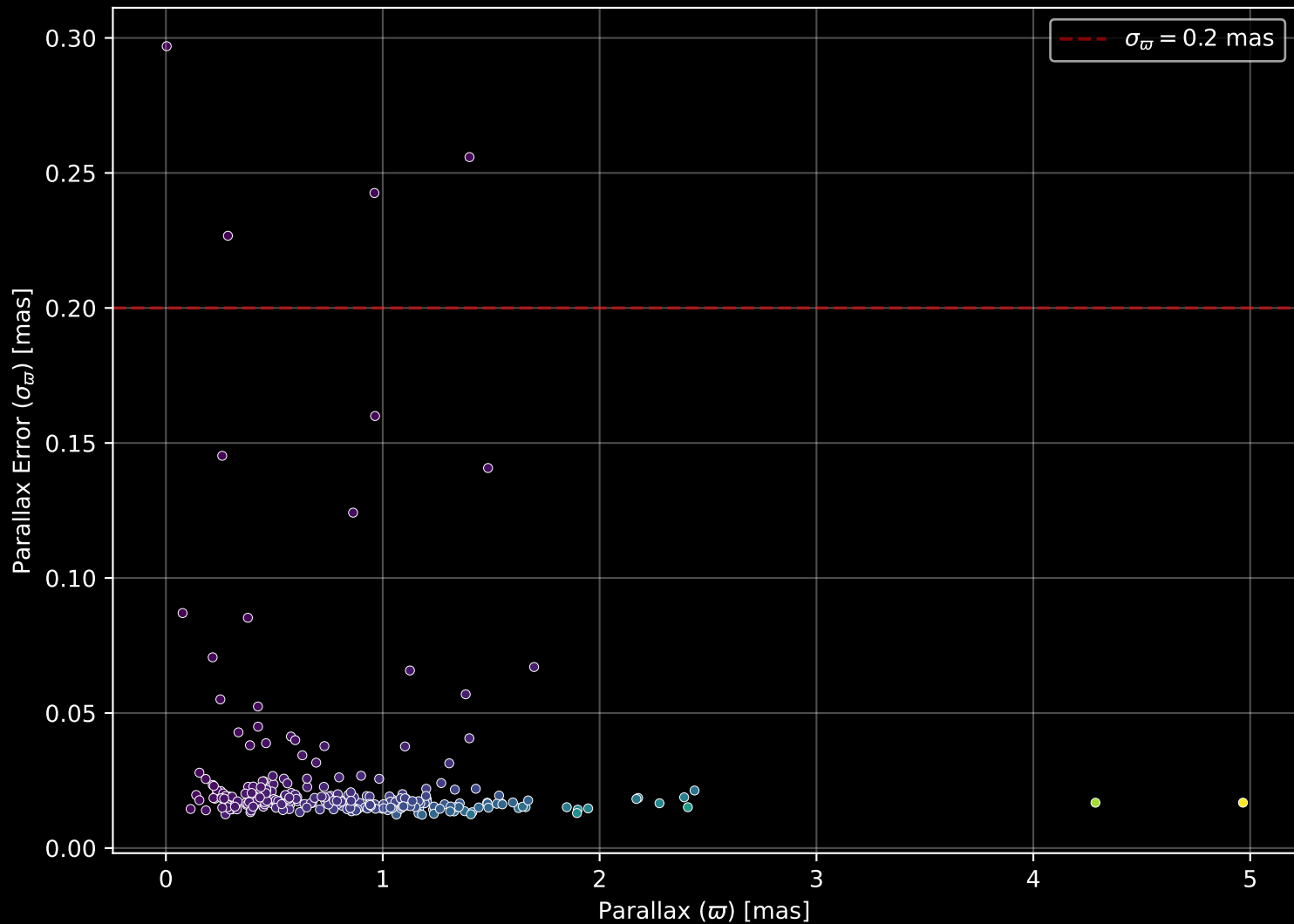
GALAH DR4 Field: [9471] Parallax Quality (n= 276)
