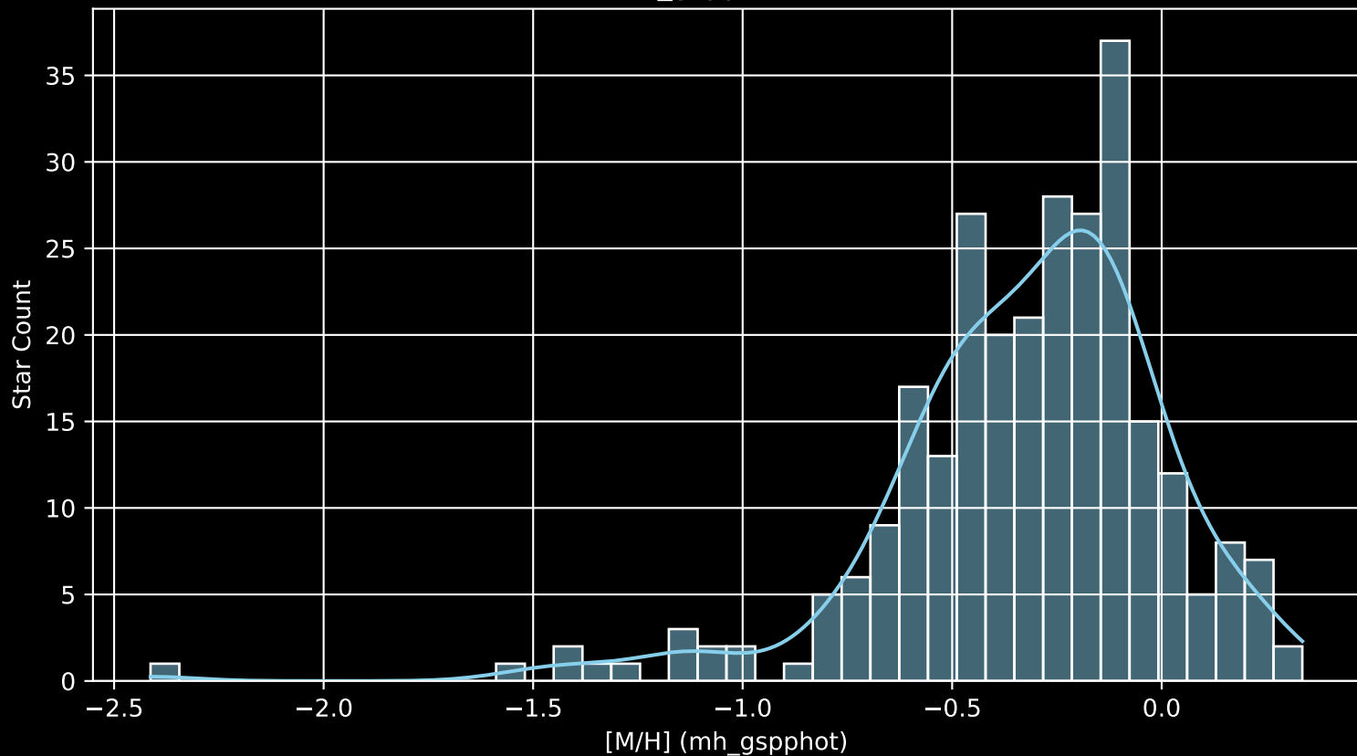
GALAH DR4 Field: [9471] [M/H] (mh_gspphot) (n= 273)
