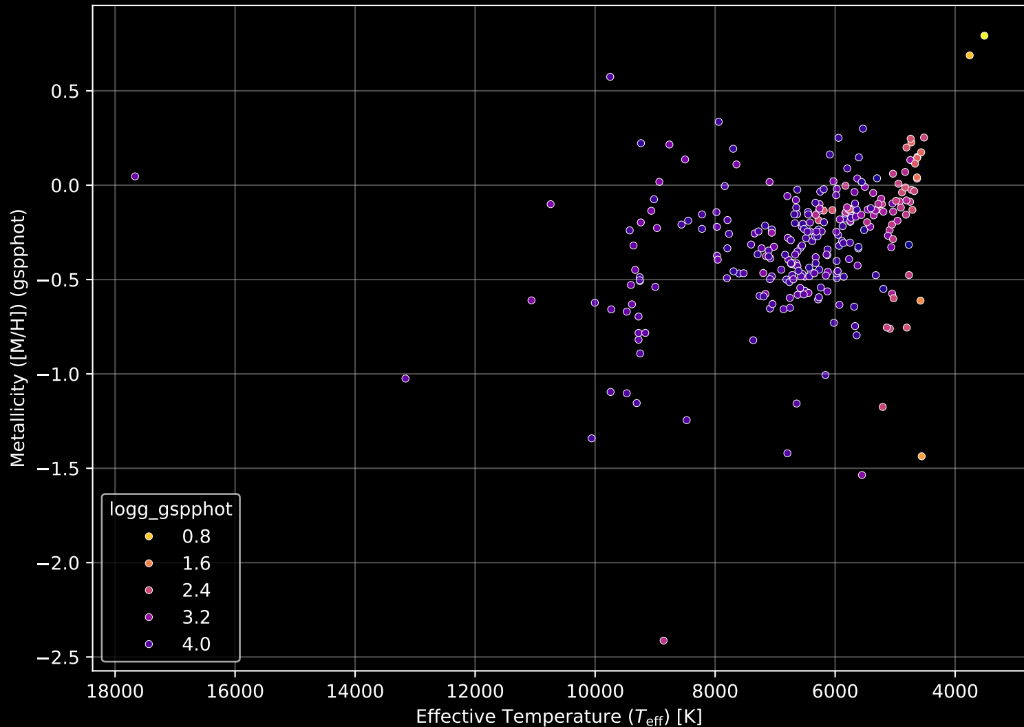
GALAH DR4 Field: [9471] Stellar Population Parameters (n= 276)
