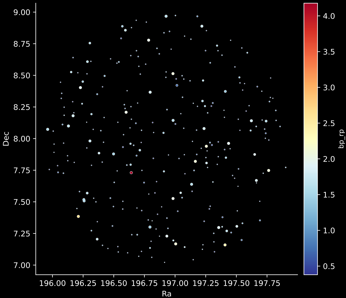
GALAH DR4 Field: [9471] Stars: 276
